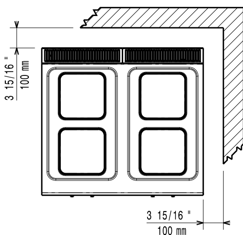
Felülnézet
